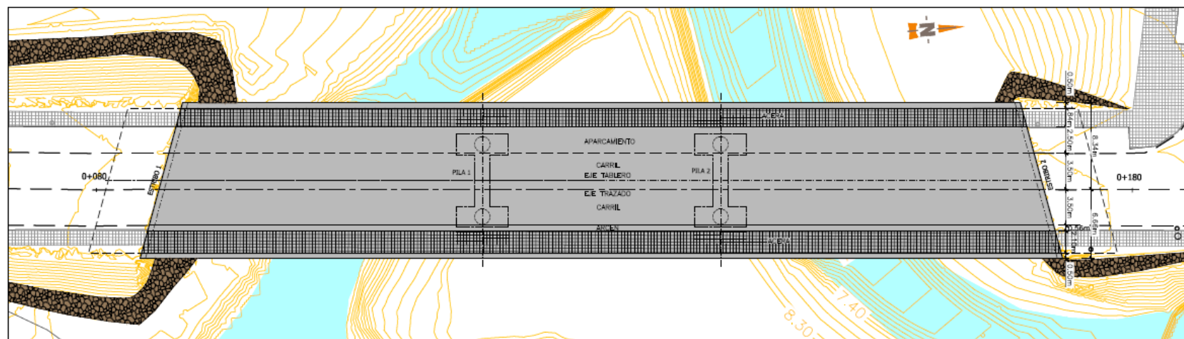
PLANTA E/1:300
