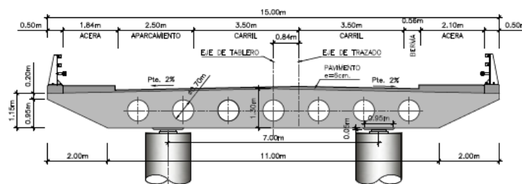
SECCIÓN TRANSVERSAL E/1:100
