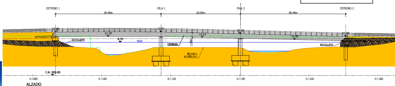
ALZADO
